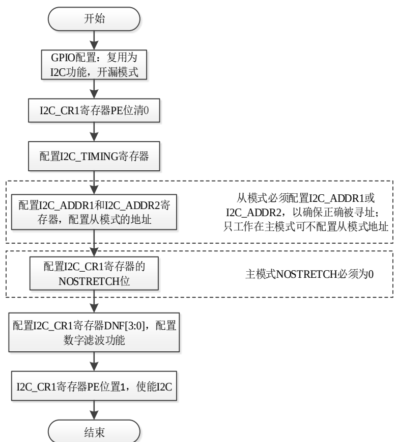
图 29-3 I2C 初始化流程
