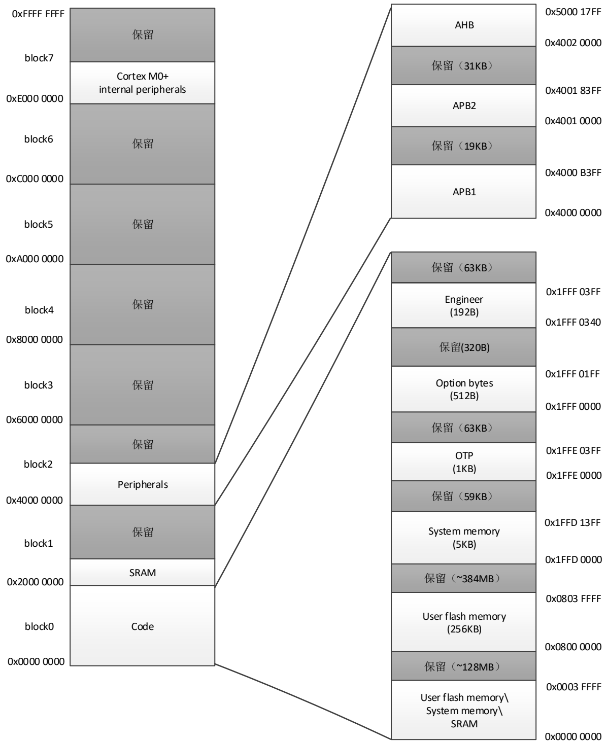
图 4-2 存储器映射
