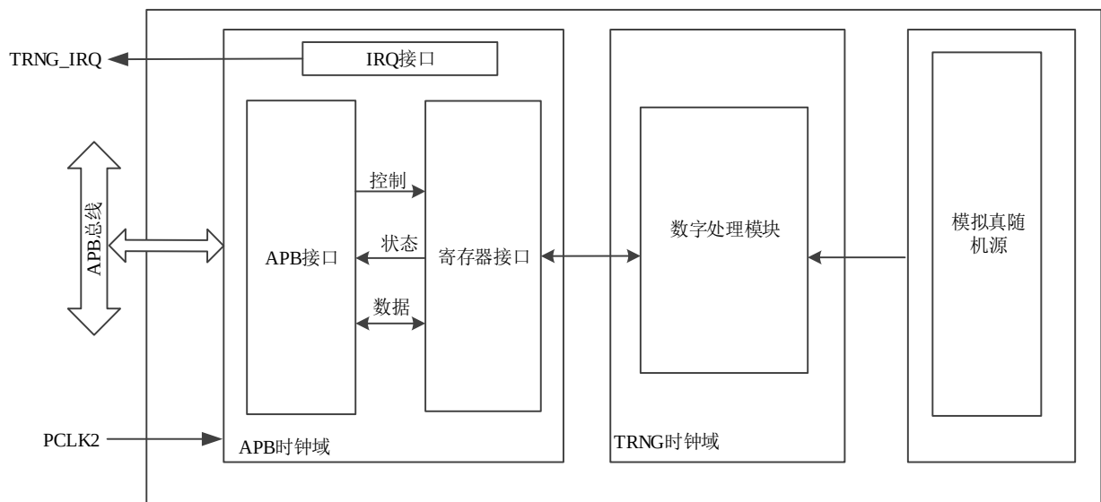
图 18-1 TRNG 框图
