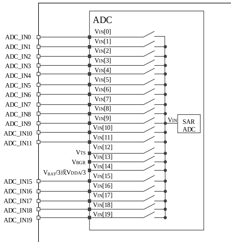
图 14-3 ADC 输入通道
