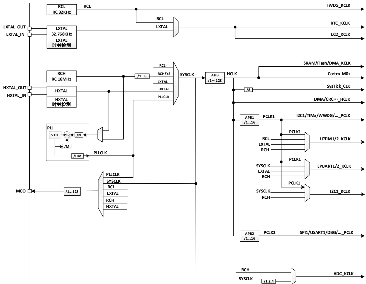
图 7-2 时钟树
