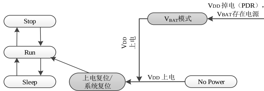
图 6-5 低功耗模式转换框图
