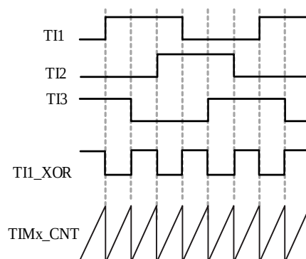
图 20-35 测量 3 个信号边沿之间的时间间隔
