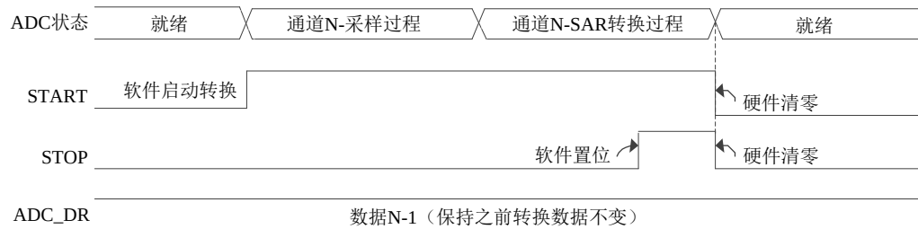
图 14-5 停止正在进行的转换
