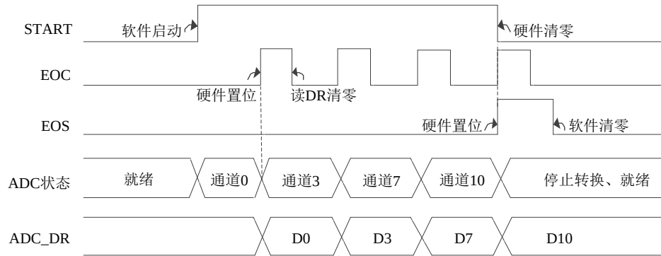
图 14-6 单次扫描转换模式，软件触发
