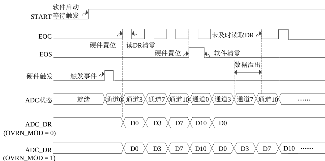
图 14-11 转换时序数据溢出处理示例 (1)
