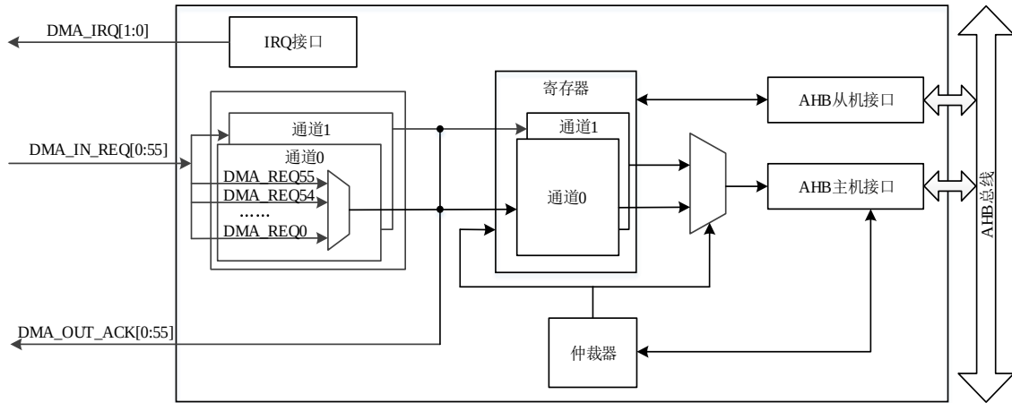
图 10-1 DMA 框图
