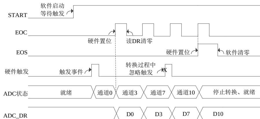
图 14-8 单次扫描转换模式，硬件触发
