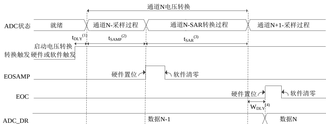
图 14-10 ADC 转换时序
