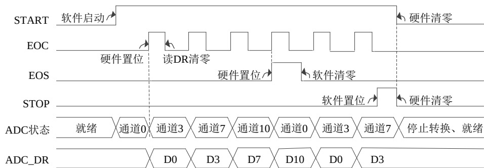
图 14-7 循环扫描转换模式，软件触发
