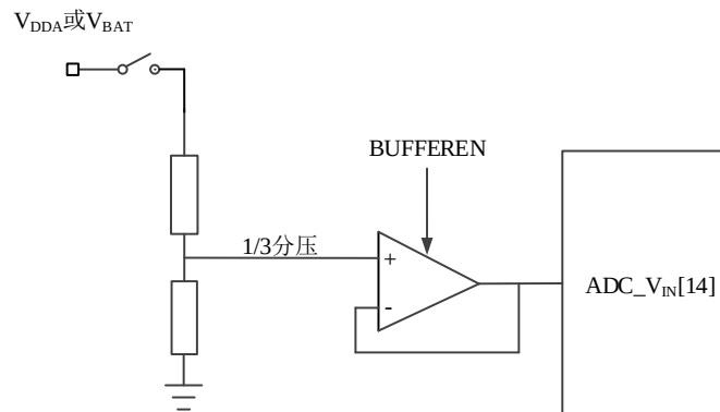
图 14-16 V_{BAT} 和 V_{DDA} 输入通道结构
