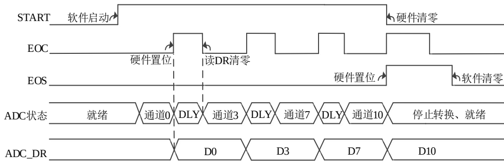
图 14-12 自动等待模式 (1)
