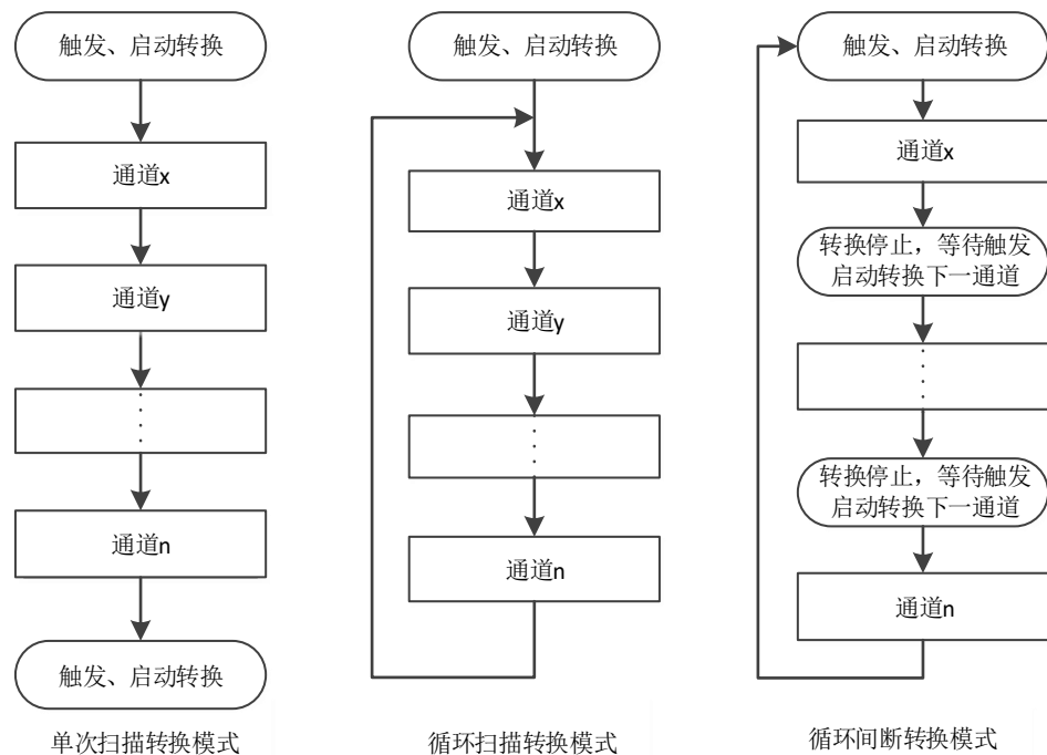
图 14-4 ADC 转换模式
