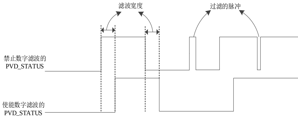
图 6-4 PVD 滤波
