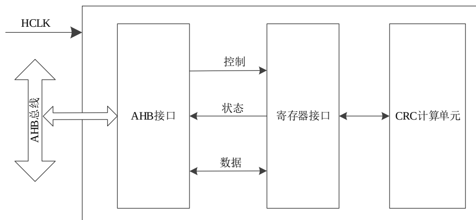
图 13-1 CRC 框图
