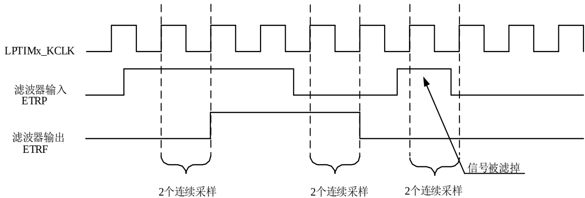
图 22-3 数字滤波时序图
