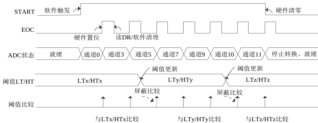
图 14-13 模拟看门狗阈值更新 (1)
