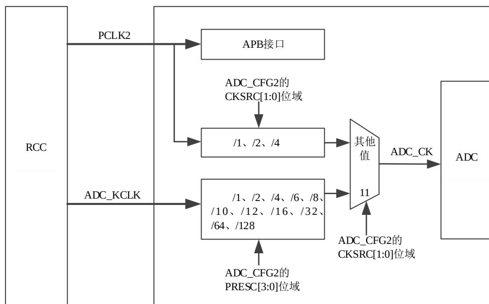
图 14-2 ADC 时钟架构 (1)
