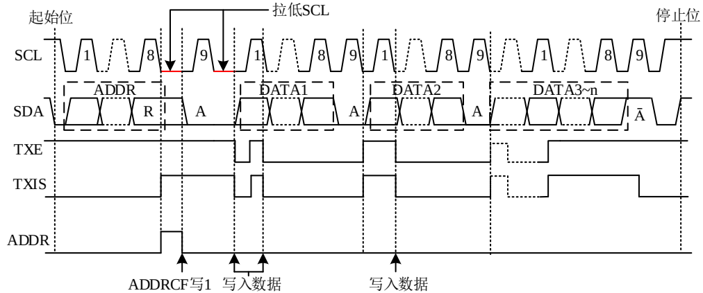
图 29-9 从模式使能时钟低电平延长发送数据
