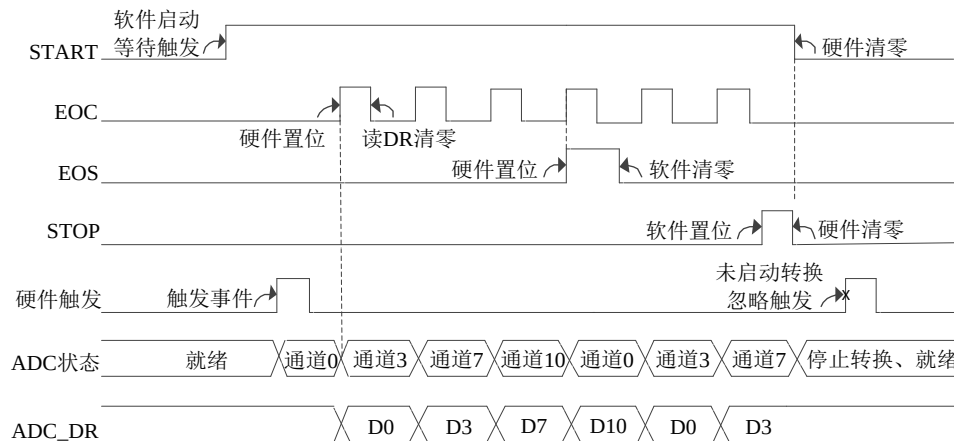
图 14-9 循环扫描转换模式，硬件触发
