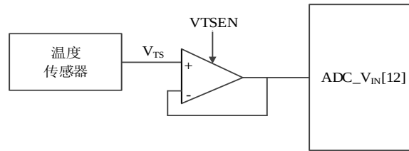
图 14-14 温度传感器输入通道结构
