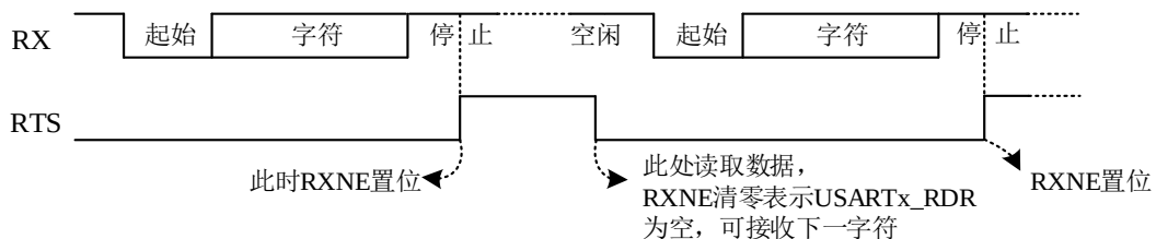
图 30-24 RTS 流控
