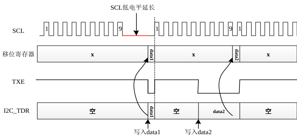
图 29-8 数据发送
