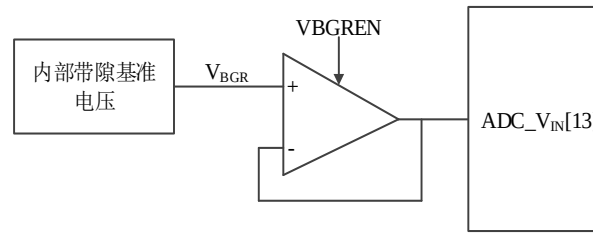
图 14-15 V BGR 输入通道结构
