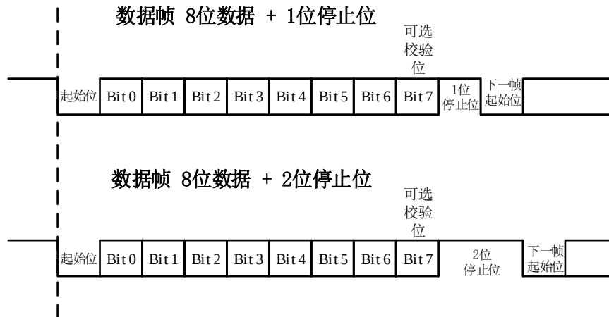
图 31-3 可编程停止位示例
